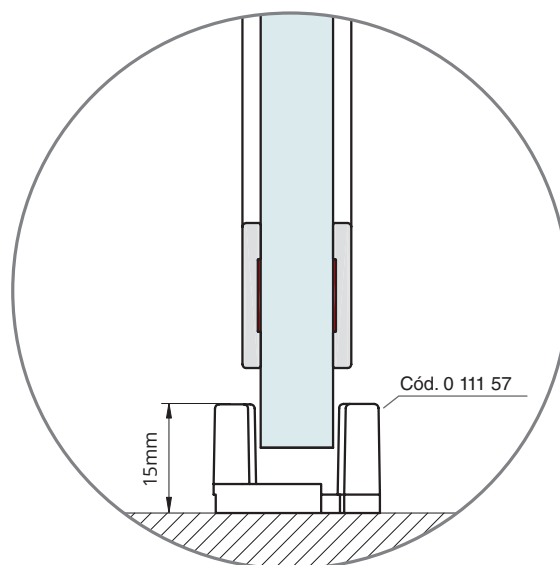
GUIADOR INFERIOR PLÁSTICO FRAME PLASTIC FRAME BOTTOM GUIDE FRAME GUIDE INFÉRIEUR PLASTIQUE
