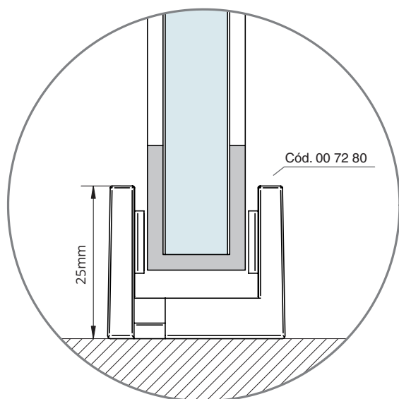
GUIADOR INFERIOR FRAME FLAT FRAME FLAT BOTTOM GUIDE GUIDE INFÉRIEUR FRAME FLAT
